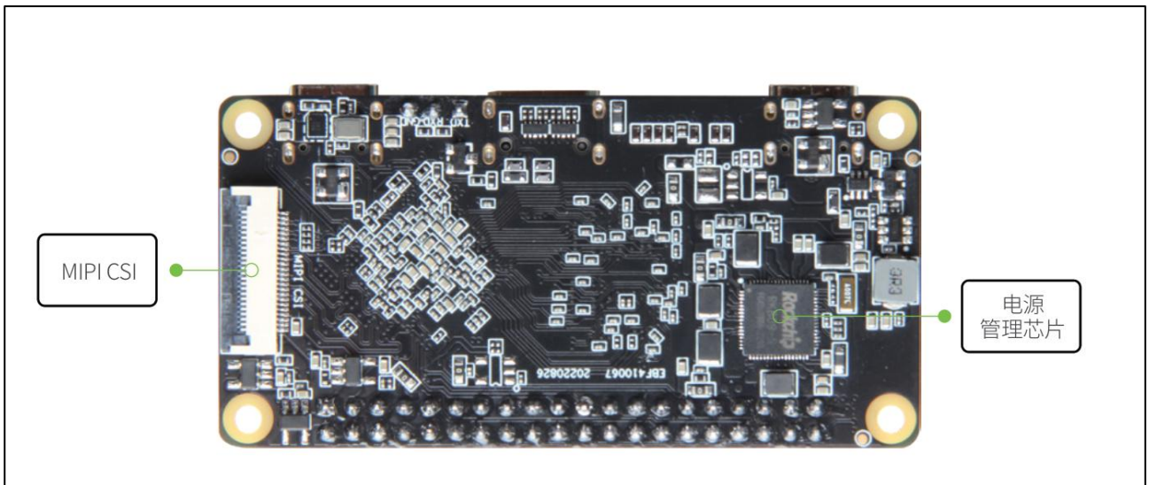
图 3.1-2 鲁班猫 Zero W 背面视图
