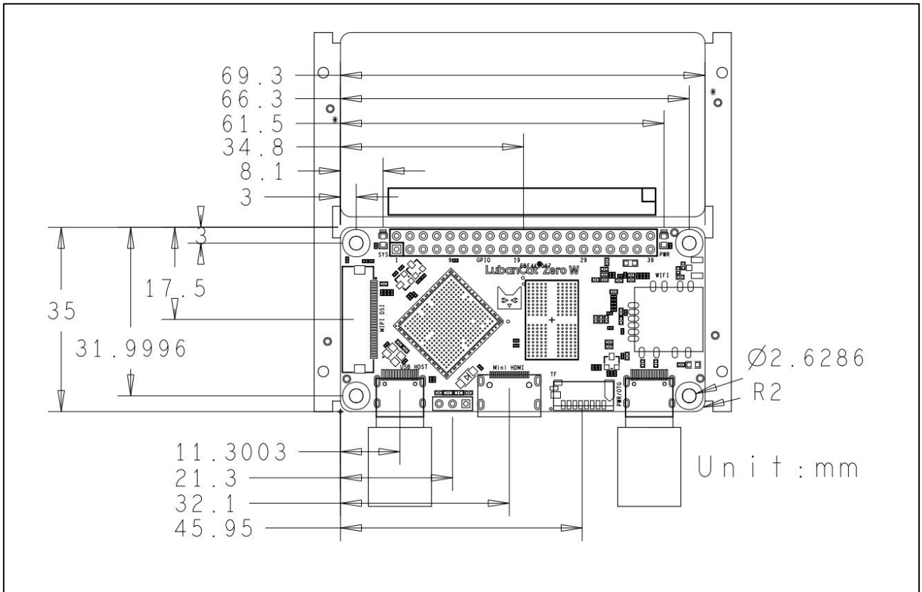
图 3.2-1 鲁班猫 Zero W 机械尺寸图
