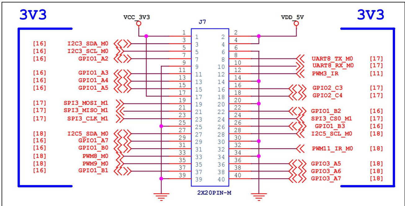
图 3.6-1 鲁班猫 Zero W 引脚原理图
