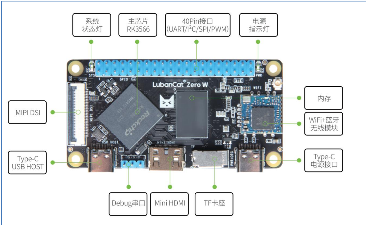
图 3.1-1 鲁班猫 Zero W 正面视图
